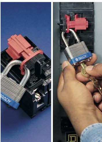
Blokkeerstanghouder
